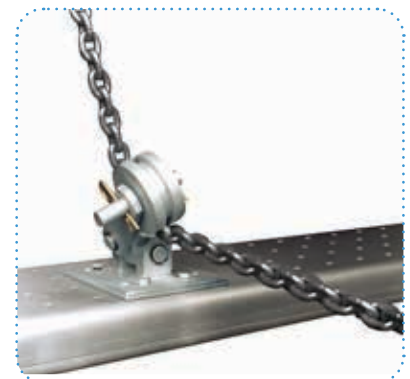
Art. 132 | Rullo rinvio per catena Pull down wheel
