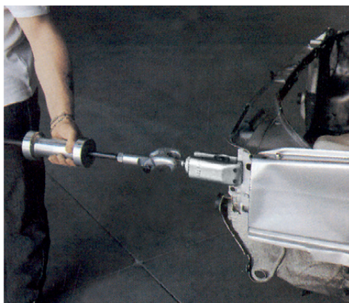
Art. 202 | Morsetto autobloccante speciale Special self locking pull clamp
